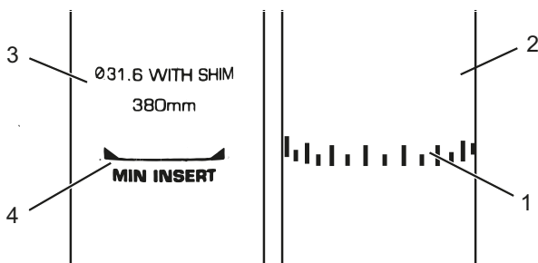
Figura 61: Vista detallada de las tijas de sillín, ejemplos de las marcas de la profundidad de inserción mínima
