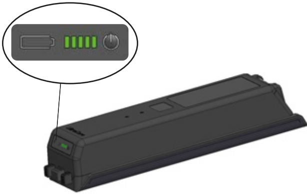
Figura 47: Posición del indicador de carga en la batería
