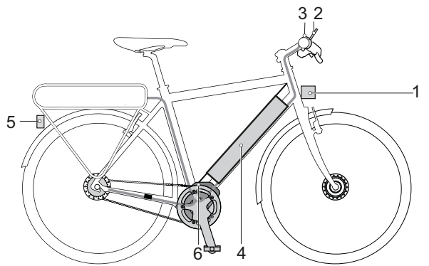
Figura 28: Esquema del sistema de accionamiento eléctrico
