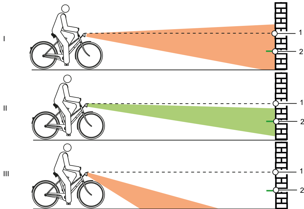
Figura 120: Luz ajustada demasiado alta (1), correctamente (2) y demasiado baja (3)
