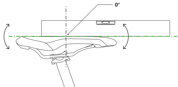
Figura 64: Inclinación del sillín horizontal con 0° de inclinación en el centro del sillín
