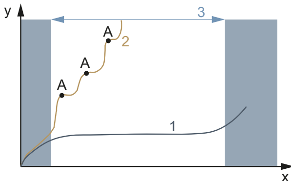
Figura 113: Diagrama de desgaste, vida útil (x) con respecto a desgaste de materiales (y)
