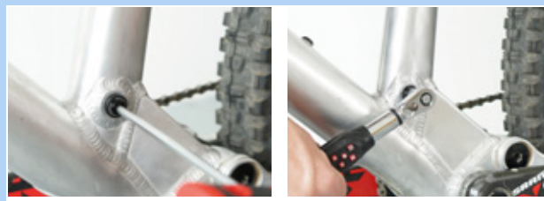
Figura 191: Atornillar la tija de sillín
