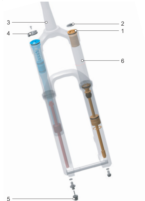
Figura 14: Estructura interna de la horquilla de suspensión neumática
